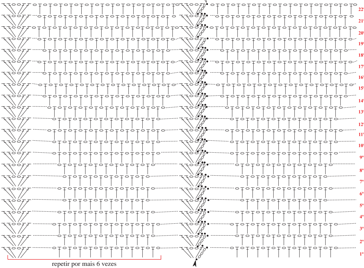
Diagrama 2- Parte inferior da peça
